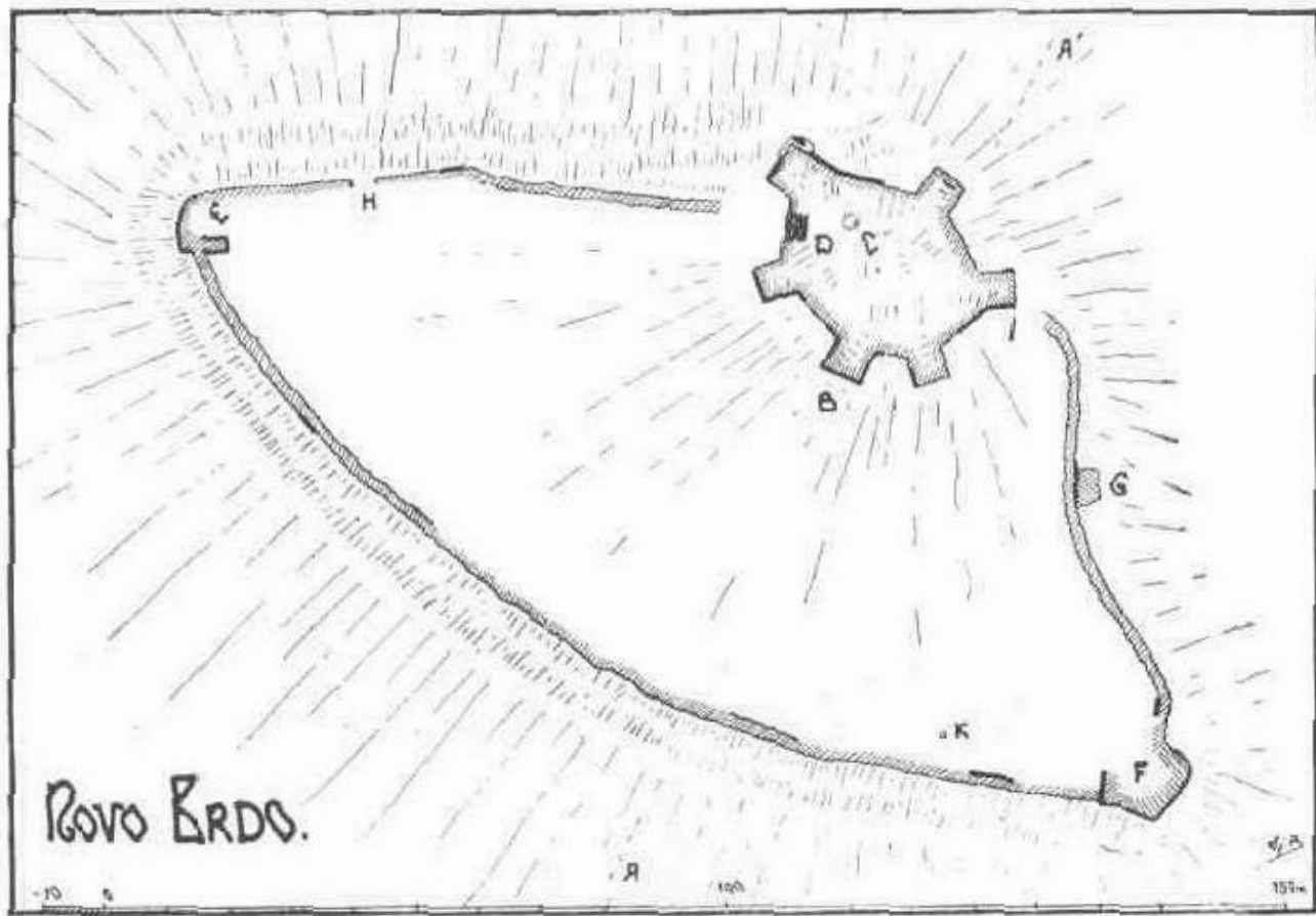
Сл. 2. — Основа Горњег и Доњег града.
