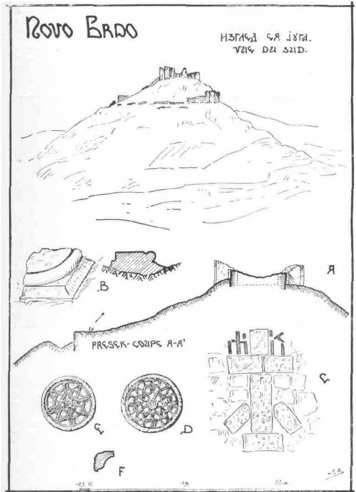
Сл. 3. — Ново Брдо: изглед, пресек и архитектонски детали.
